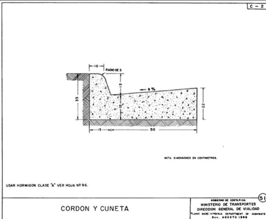
Imagen N°1. Sección transversal cuneta y cordón de caño.
