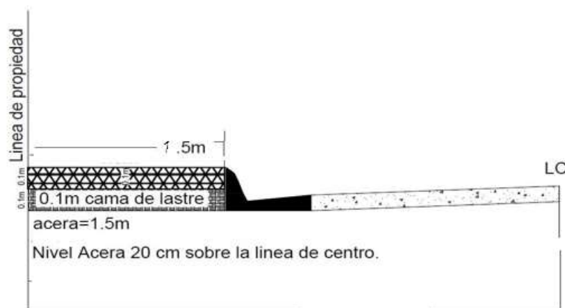
Imagen N°2- Detalle para construcción de Acera.
